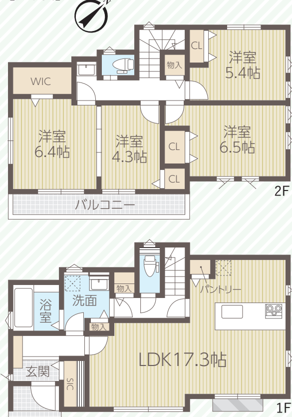
【間取図】
